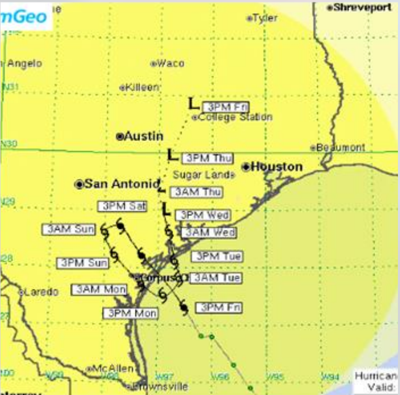
8/25 Track
